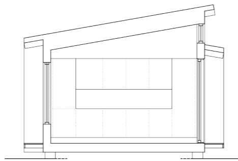
SEKTION A-A
