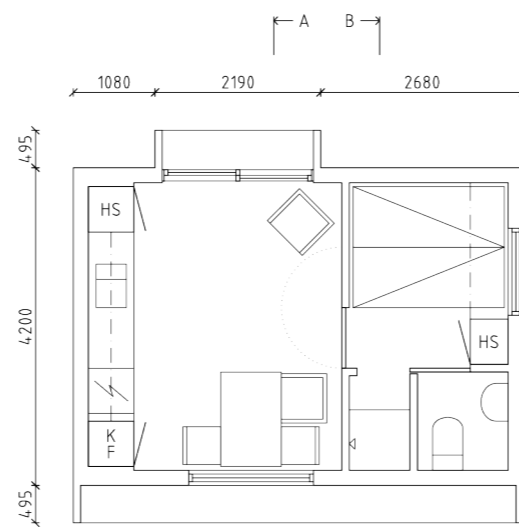
ENTRÉPLAN
